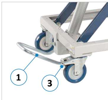
Figure 6 : étrier de pied et frein
