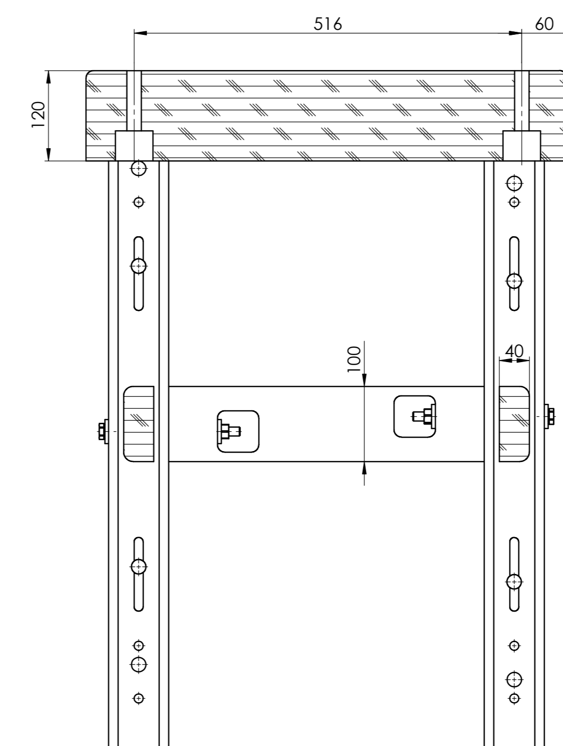
REZ A-A MÉRITKO 1 : 5
